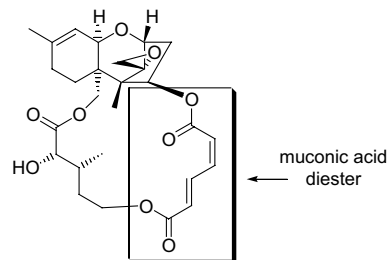
Figure 1. Verrucarins A.
